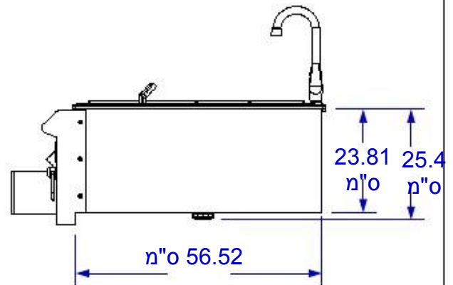
מבט צד ימני
